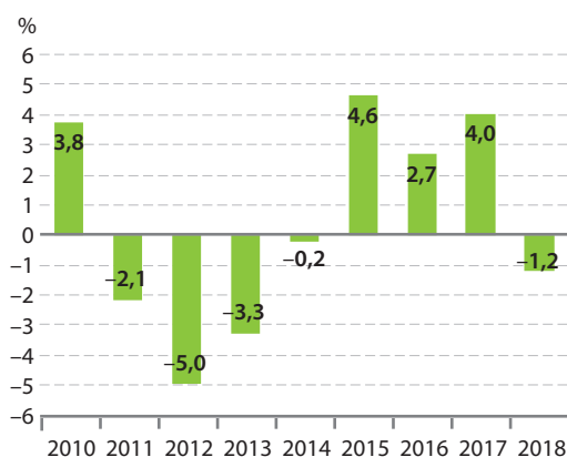
6.5. ábra Magyarország teljes energiafelhasználásának változása az előző évhez képest
