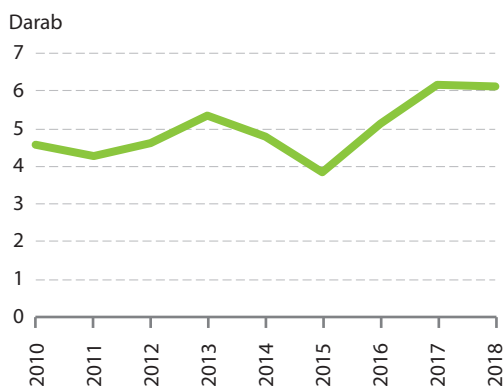
6.4. ábra A tíz kilométer ivóvízvezetékre jutó csőtörések számának alakulása
