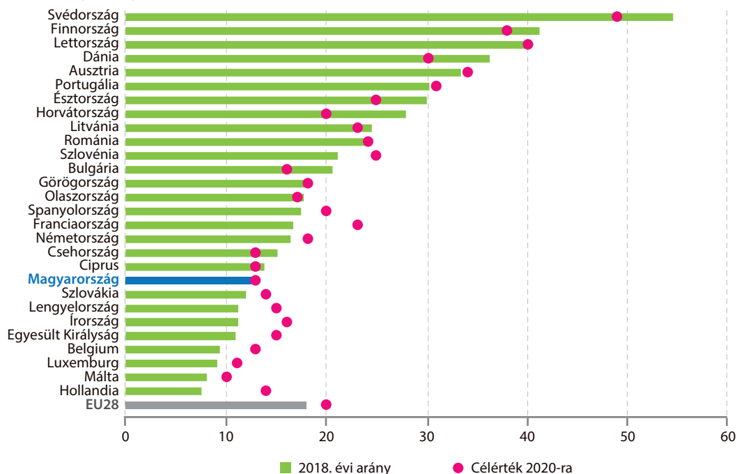
6.6. ábra A megújuló energiaforrások részesedése a teljes energiafelhasználásból az uniós tagországokban
