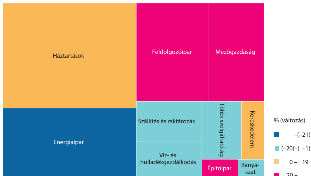
6.1. ábra Nemzetgazdasági ágak és háztartások üvegházhatásúgáz-kibocsátásának megoszlása 2017-ben, és a kibocsátás változása 2010-hez képest
