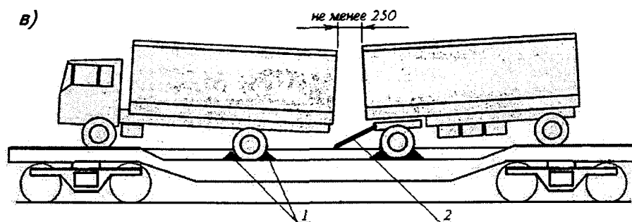
Рисунок 13 – Размещение и крепление автопоезда (автомобиль-прицеп)
