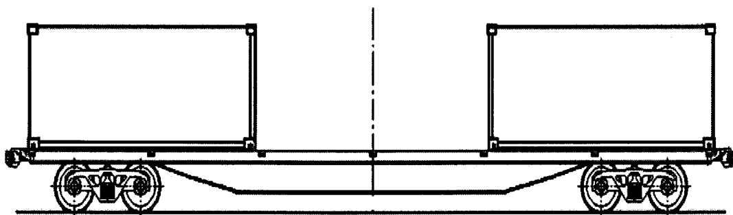
12. ábra - Kettő darab 20 láb hosszúságú konténer elhelyezése a 13900 mm, 14400 mm és 14720 mm forgócsap távolságú nagykonténer-szállító pórekocsik homlokrészeinél
