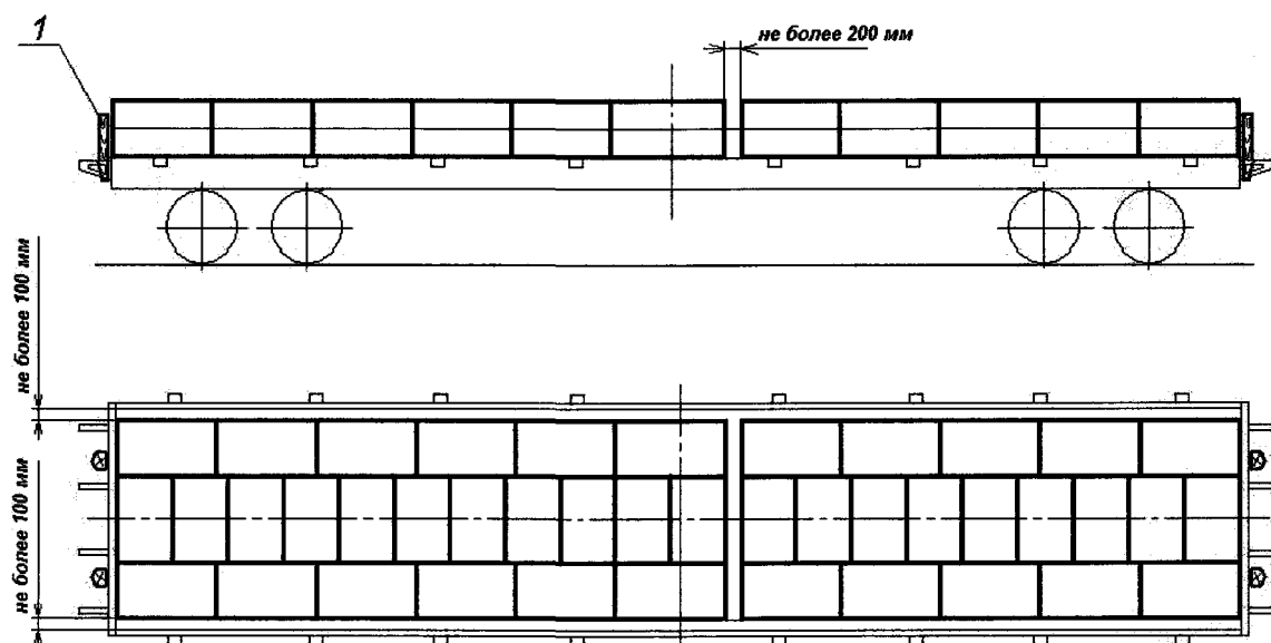
Рисунок 8 – Принципиальная схема размещения и крепления пакетов на платформе
