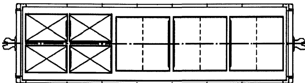
5. ábra - A konténerek elrendezése konténerszállító kocsiban, kívülről a sarokrakoncákhoz erősített gerendakapocs vagy gerenda homlokbiztosítással
