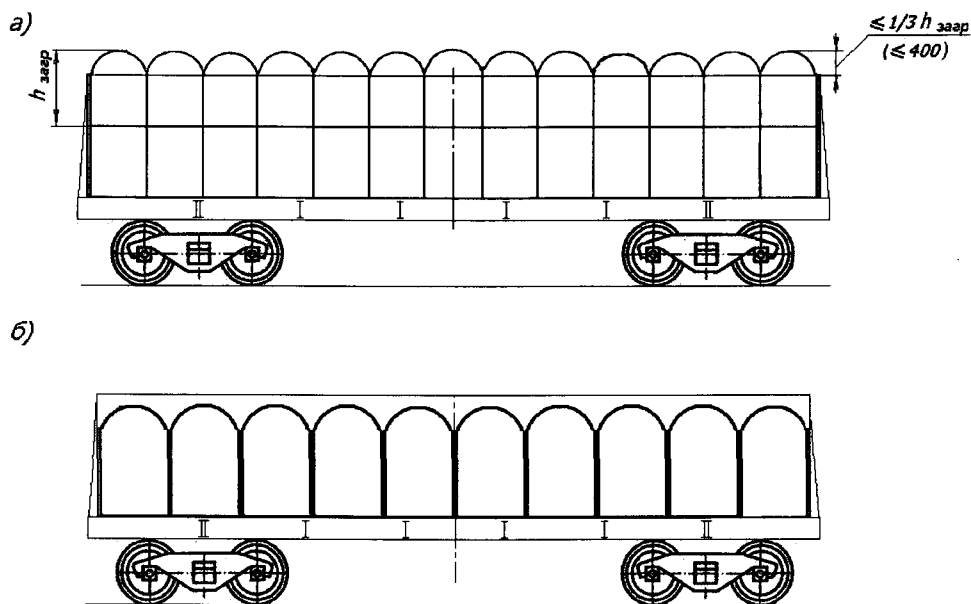
Рисунок 28 – Принципиальная схема размещения мягких контейнеров в полувагоне в один или два яруса по высоте
