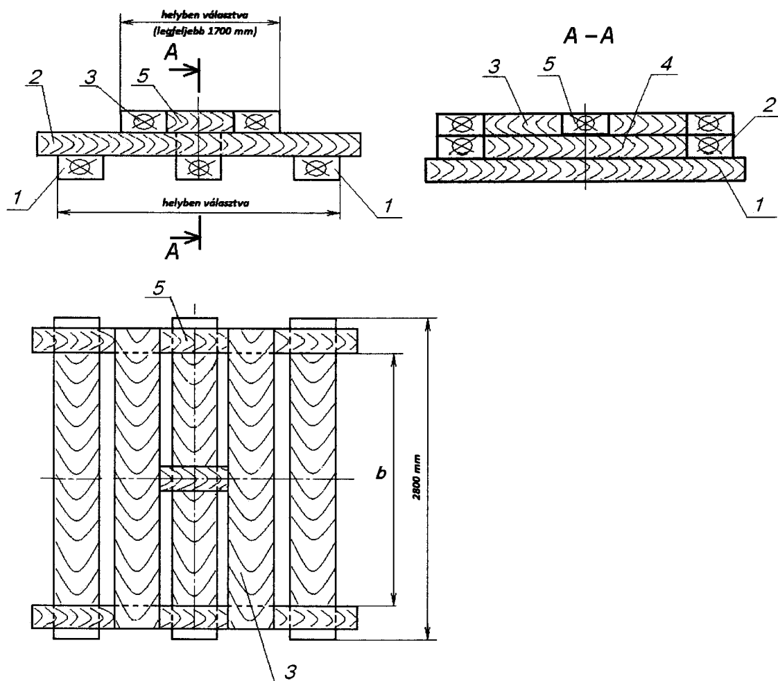
8. ábra A támasztókeret
