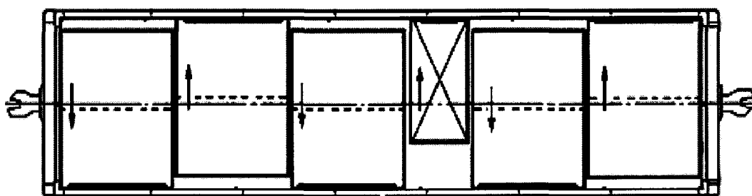
2. ábra - A konténerek elrendezése 12228 mm belső szekrényhosszúságú, magas oldalfalú teherkocsiban és konténerszállító kocsiban
