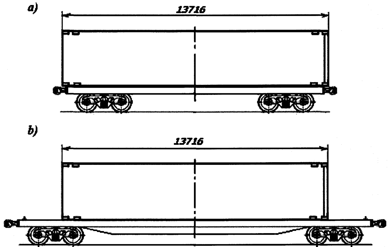
16. ábra - A 45 láb hosszúságú konténer elhelyezése a nagykonténer szállító pórekocsiban: a - 9720 mm forgócsap távolság esetén; b - 13900 mm, 14400 mm és 14720 mm forgócsap távolság esetén
