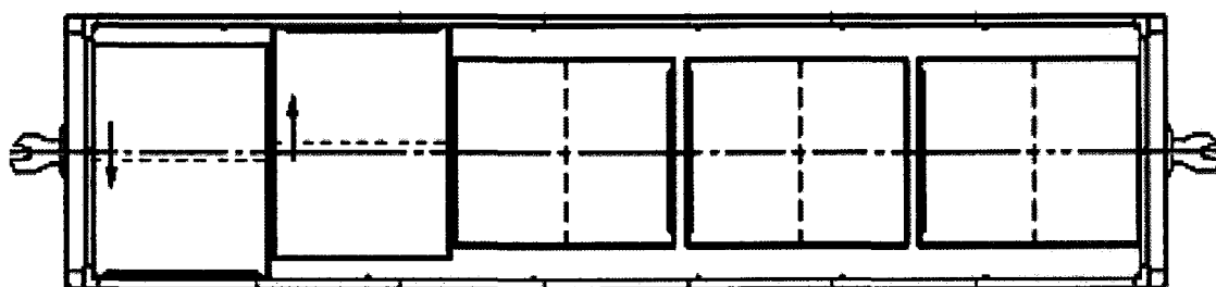
3. ábra - A konténerek elrendezése 12324 mm belső szekrényhosszúságú, magas oldalfalú teherkocsiban és konténerszállító kocsiban
