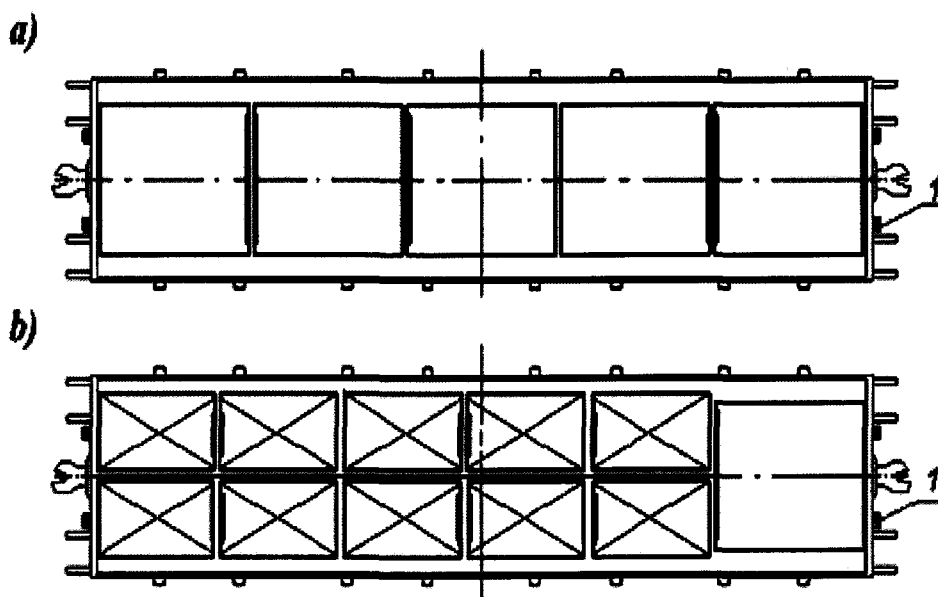
1. ábra - A konténerek elrendezése 13300 mm belső szekrényhosszúságú, általános rendeltetésű pórekocsiban 1 - homlokrakonca
