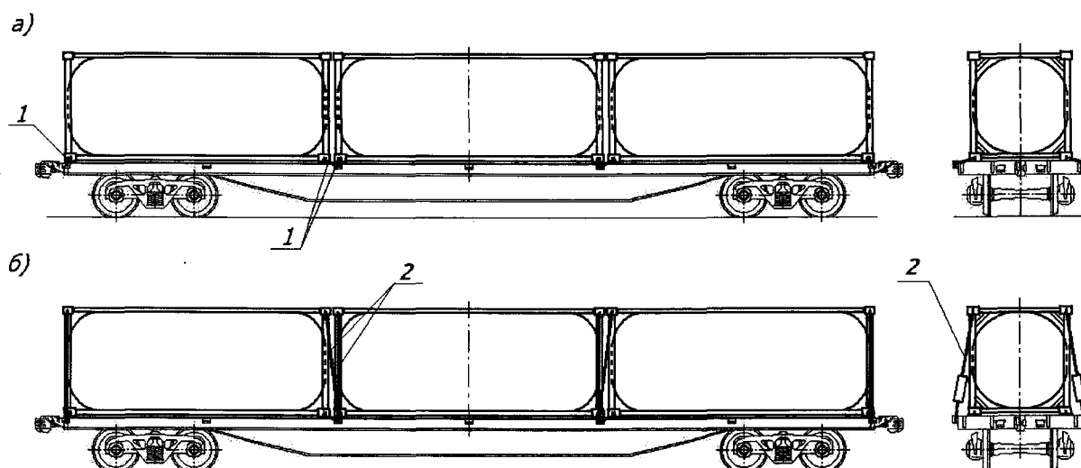
Рисунок 26-8 – Дополнительное крепление контейнеро-цистерн на платформе для крупнотоннажных контейнеров:
