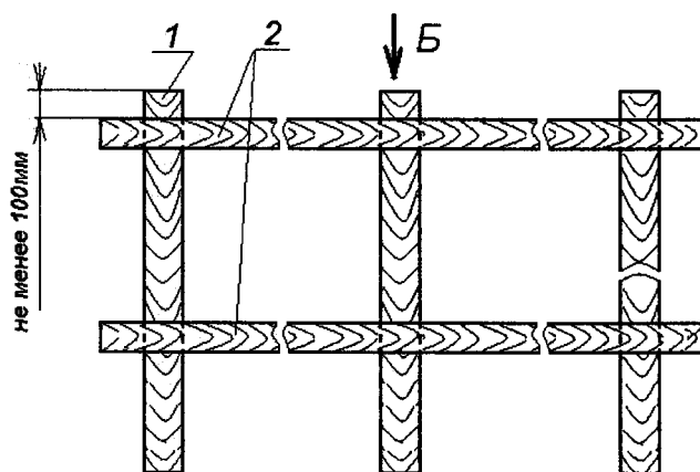
Рисунок 7 – Варианты изготовления распорного щита 1 – стойка; 2 – упорная доска
