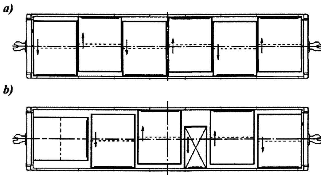
4. ábra - A konténerek elrendezése 12690-12750 mm belső szekrényhosszúságú, magas oldalfalú teherkocsiban
