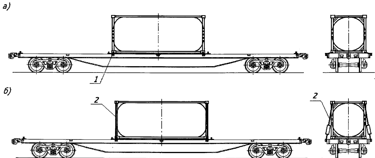
26-10. ábra – Tankkonténerek kiegészítő lekötése a pórekocsin nagykonténerek esetén
