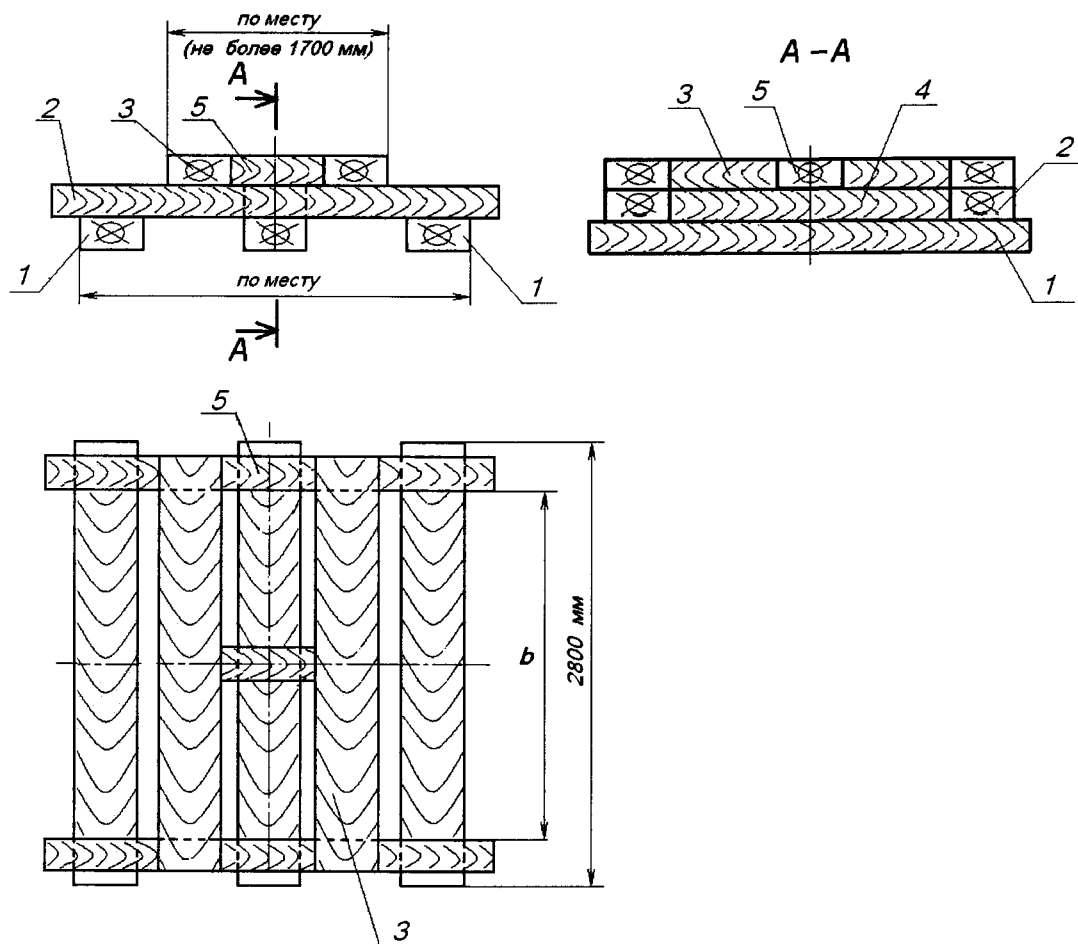
Рисунок 8 – Распорная рама
