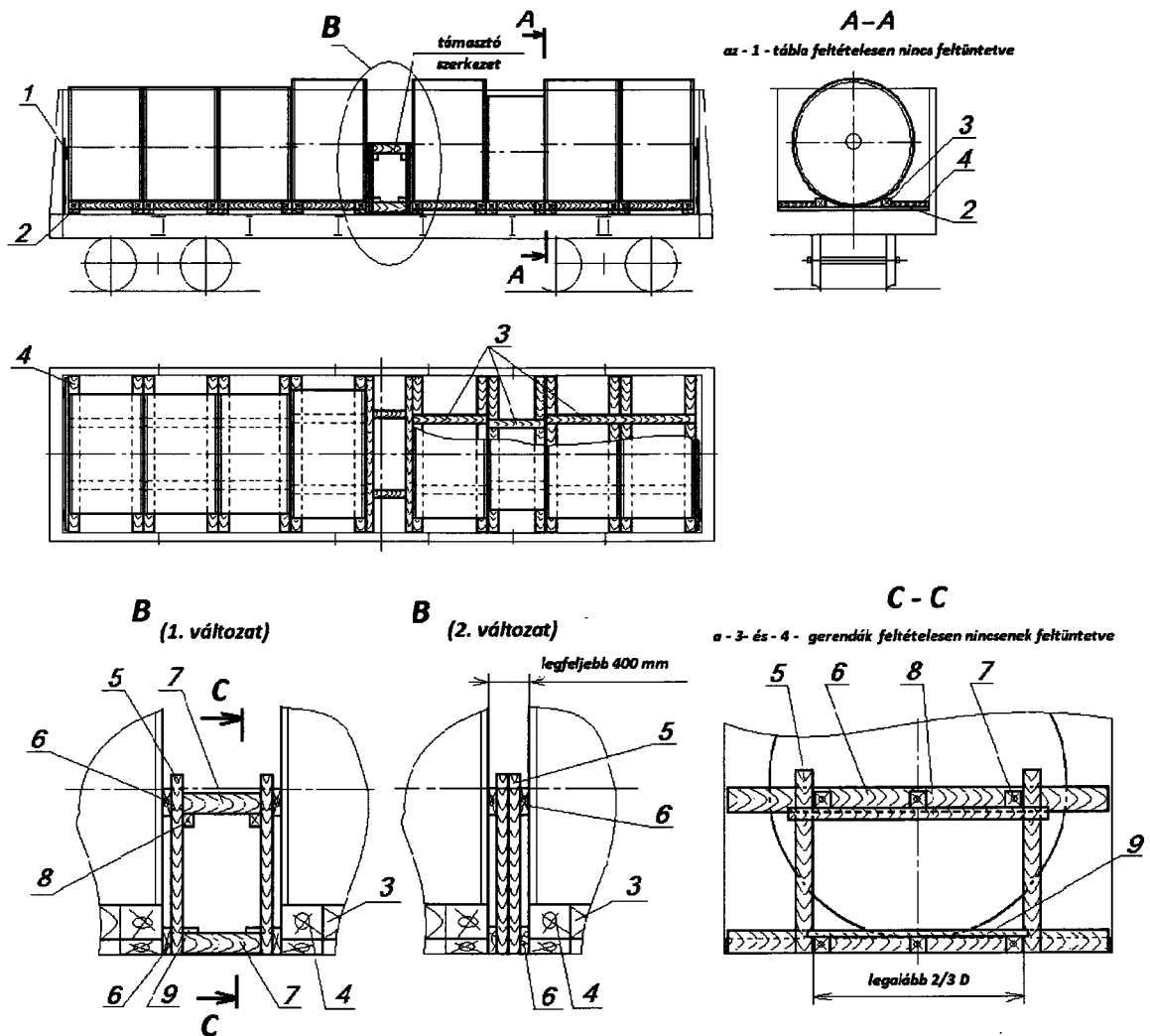
9. ábra 1 – tábla; 2 – alátétfa; 3 – támfa; 4, 7 – távtartó fabetét; 5 – oszlop; 6 – támdeszka; 8 – alátámasztó betétfa ; 9 – összekötő lap
