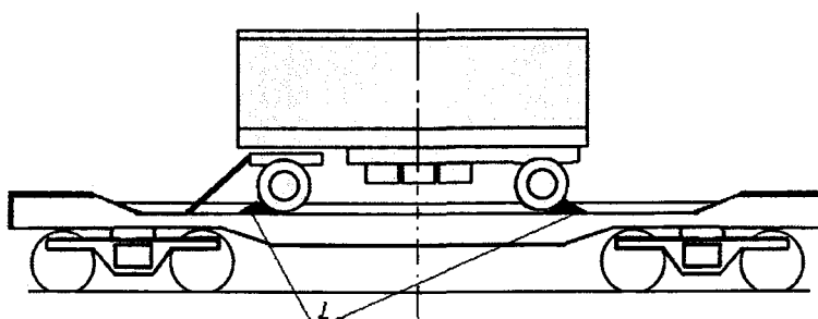
Рисунок 15 – Размещение и крепление прицепа
