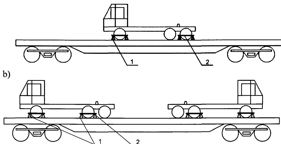
10. ábra A nyerges vontatók elhelyezése és biztosítása 1 – kerékelőtét; 2 – oldaltám
