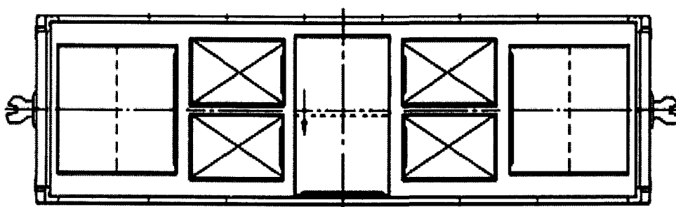
6. ábra - A konténerek elrendezése konténerszállító kocsiban, belülről a sarokrakoncákhoz erősített támgerenda homlokbiztosítással
