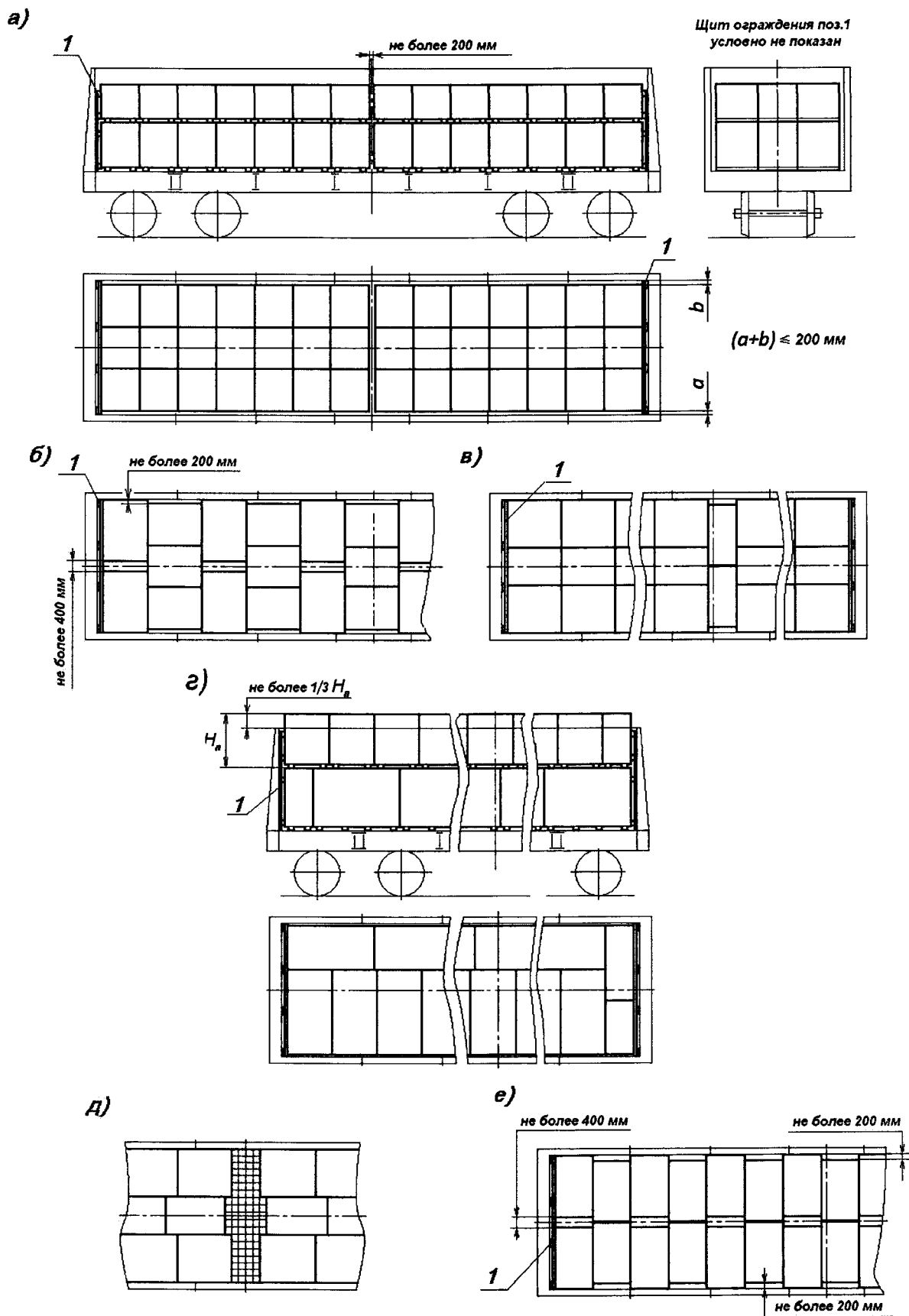
Рисунок 3 – Примеры размещения пакетов
