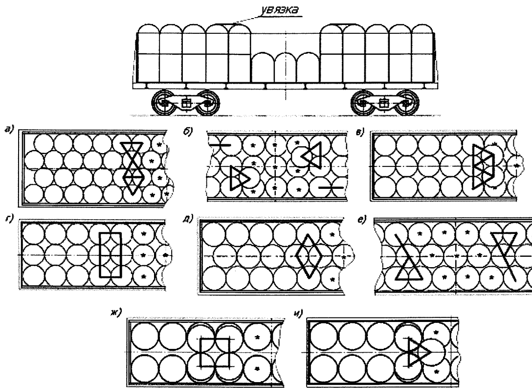
Рисунок 30 – Размещение мягких контейнеров во втором ярусе * – обозначение контейнеров, размещенных в первом ярусе
