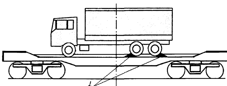
Рисунок 14 – Размещение и крепление автомобиля
