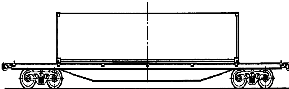
15. ábra - Egy darab 40 láb hosszúságú konténer elhelyezése a 13900 mm, 14400 mm és 14720 mm forgócsap távolságú nagykonténer-szállító pórekocsiban
